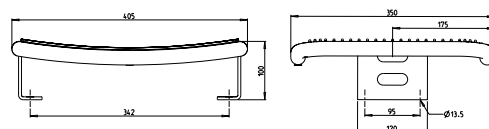
Für Mauer, Art.-Nr.: 51408
