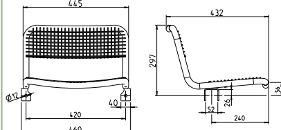
Für Zarge 50x50 mm, Art.-Nr.: 52306
