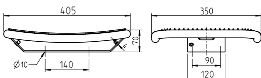
Mit Adapter Olympia, Art.-Nr.: 53223
