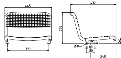
Erlau Standard für Mauer und Zarge, Art.-Nr.: 53710
