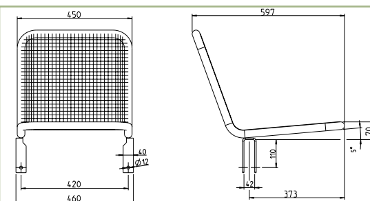
Für Zarge 100x40 mm, Art.-Nr.: 51002
