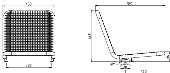
Erlau Standard für Mauer und Zarge, Art.-Nr.: 53696
