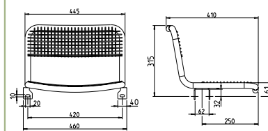
Für Zarge 60x60 mm, Art.-Nr.: 54012
