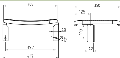
Für Zarge 100x40 mm, Art.-Nr.: 53235
