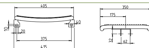
Für Zarge 60x60 mm, Art.-Nr.: 54011
