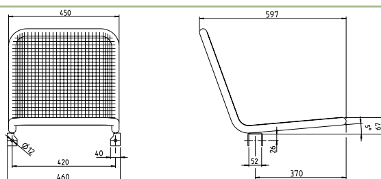
Erlau Standard für Mauer und Zarge, Art.-Nr.: 53696
