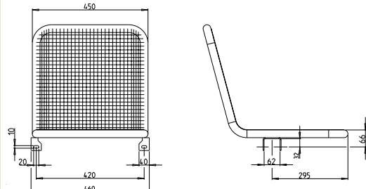
Für Zarge 60x60 mm, Art.-Nr.: 54010
